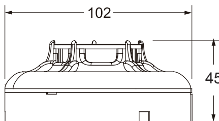
尺寸圖
