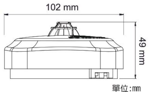
尺寸圖
