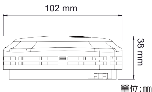
尺寸圖
