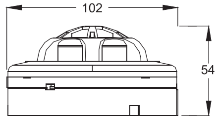
尺寸圖
