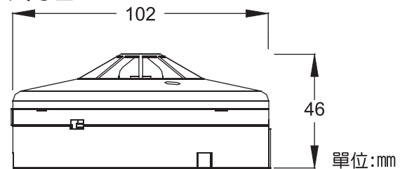
尺寸圖
