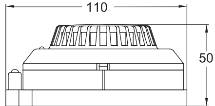
尺寸圖
