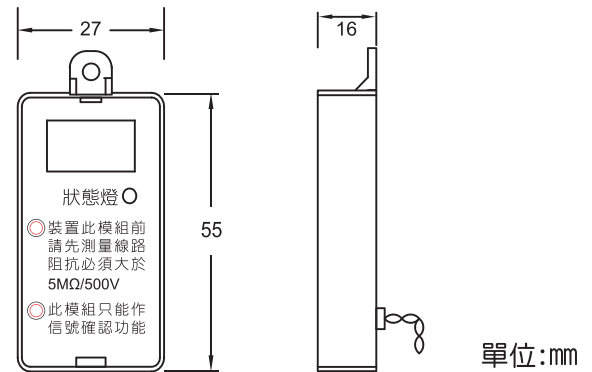
尺寸圖
