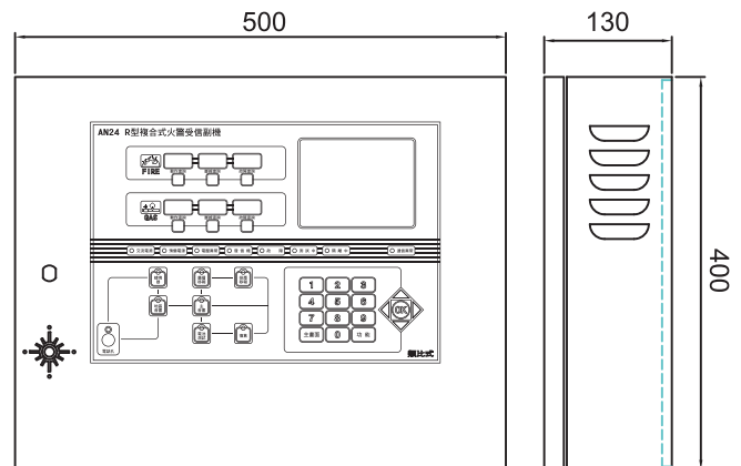
尺寸圖
