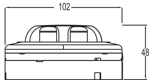
尺寸圖
