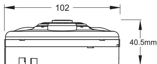
尺寸圖
