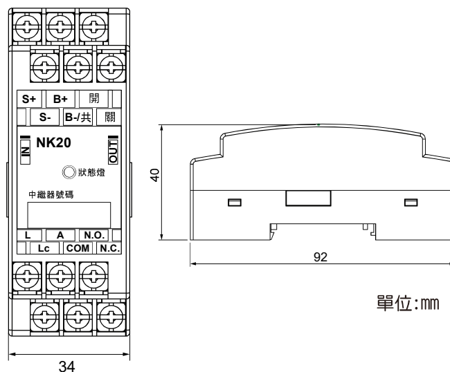
尺寸圖
