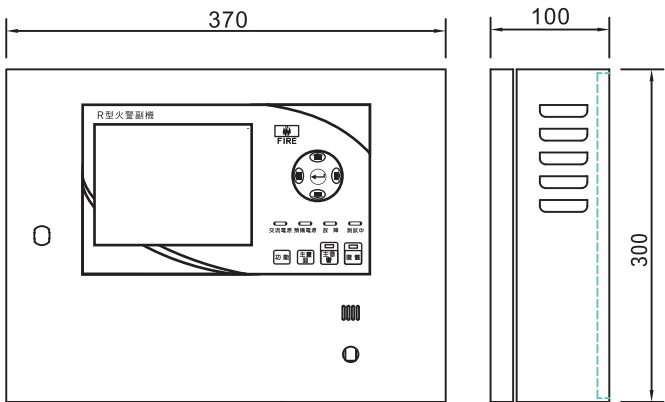
尺寸圖
