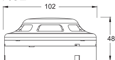
尺寸圖
