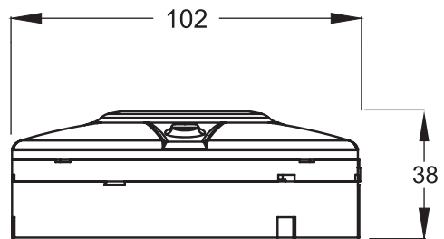
尺寸圖
