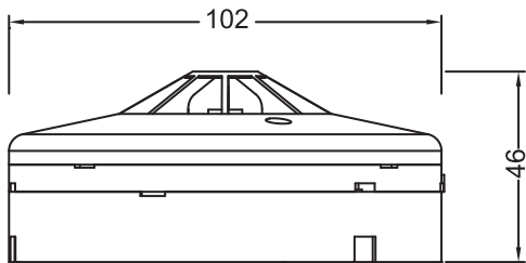
尺寸圖
