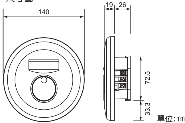
尺寸圖
