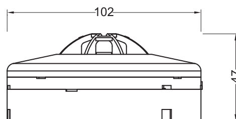
尺寸圖
