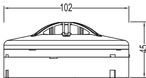
尺寸圖
