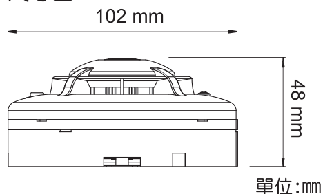
尺寸圖
